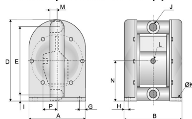
Насосы серии T из нержавеющей стали
