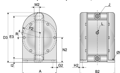
Бочковые насосы TD
