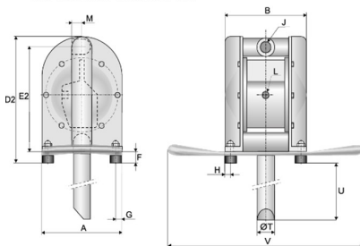
Насосы с двойными патрубками TT
